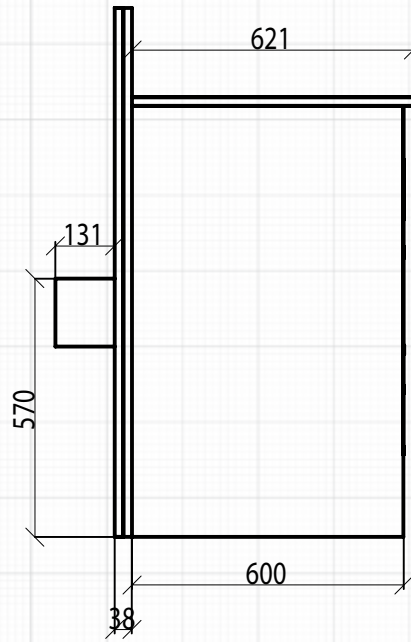
Seitenansicht
