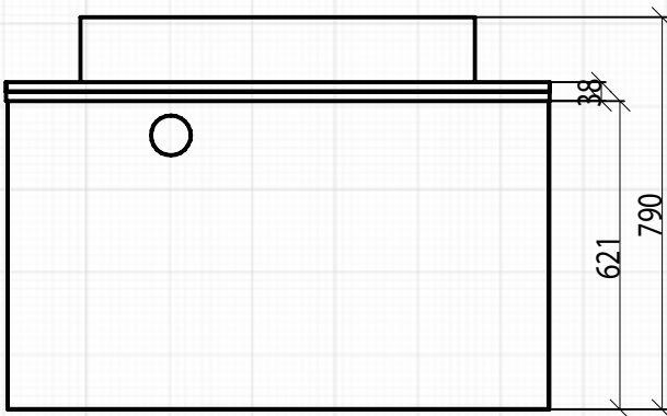
Aufsicht
