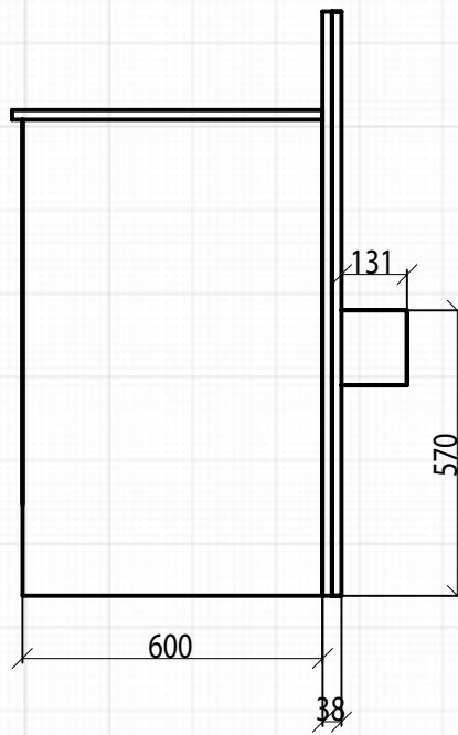
Seitenansicht
