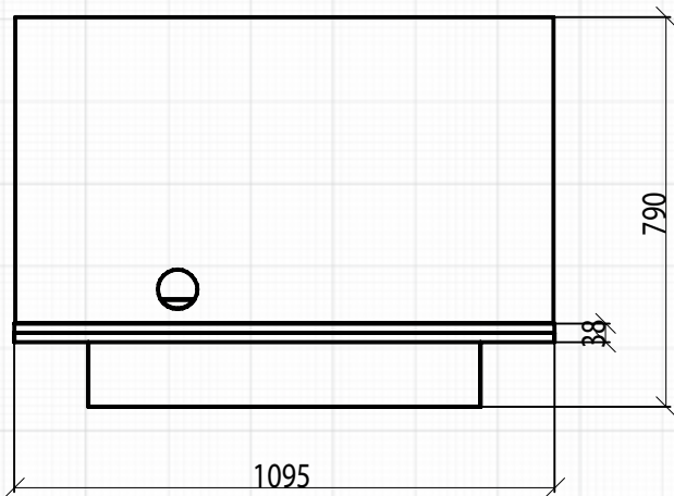
Aufsicht
