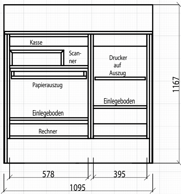
Rückansicht
