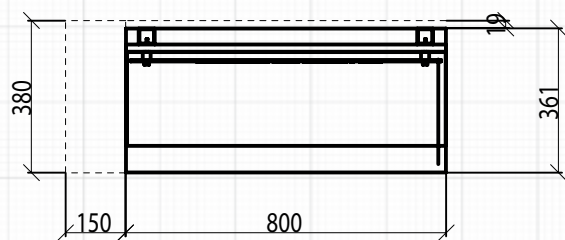
Aufsicht
