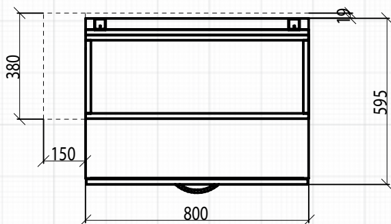
Aufsicht
