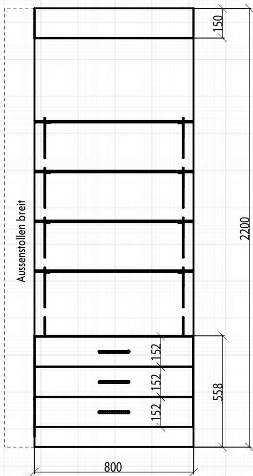
Frontansicht
