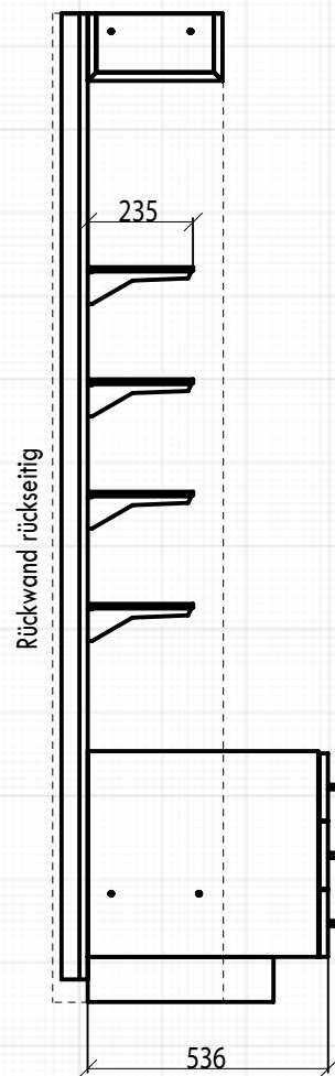
Seitenansicht
